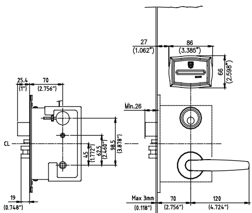
* Cerradura embutir EURO
