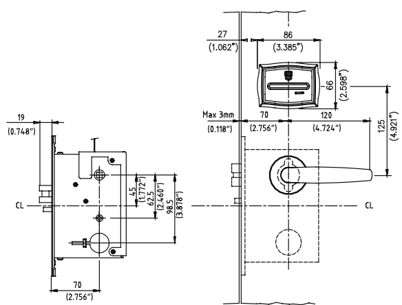
* Cerradura embutir AUS
