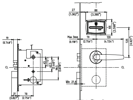
* Cerradura embutir JPN
