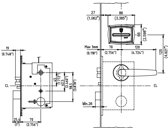
* Cerradura embutir ANSI
