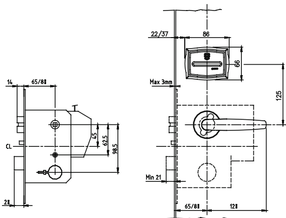
* Cerradura embutir EURO
